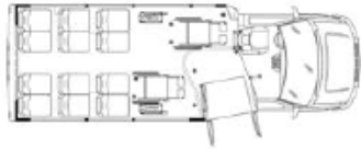
24', 12+4 Passenger, 2 w/c
